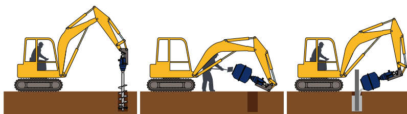
Forage, mélange et remplissage avec une excavatrice.
