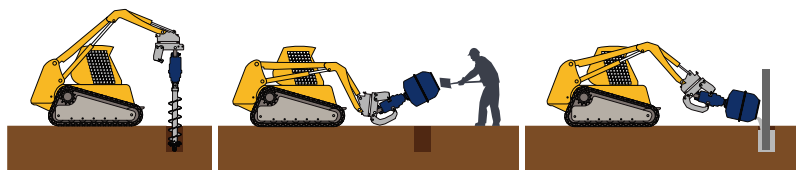
Forage, mélange et remplissage avec une chargeuse compacte.
